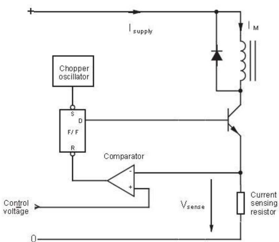
Схема с едно захранващо напрежение
